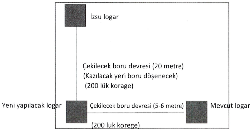
Şekil 3.1. Konak iskelesinde (Pasaport tarafı) yapılacak pis su devresi tadilatı resmi
